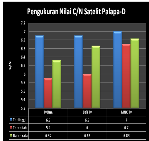
Gambar 5 Pengukuran Nilai C/N Satelit Palapa D
